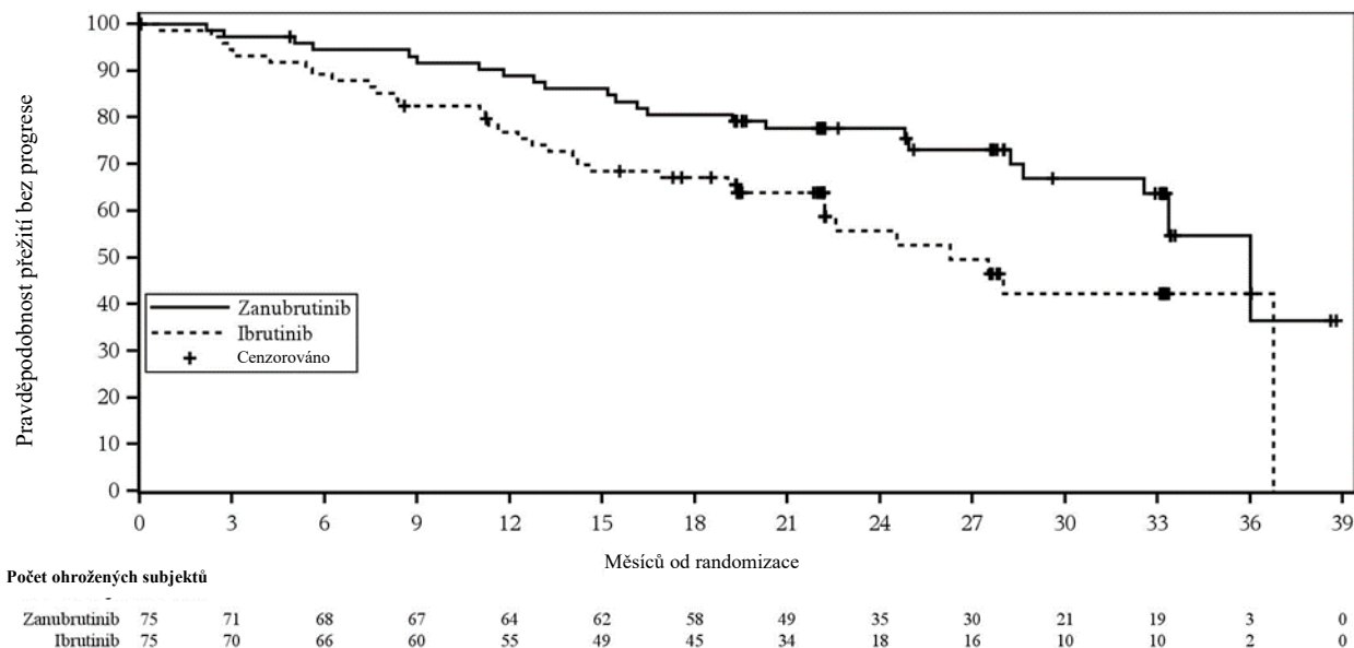
Obrázek 3: Kaplanova-Meierova křivka přežití bez progresce podle nezávislého centrálního hodnocení u pacientů s mutací del(17p) nebo TP53 (ITT) (datum ukončení sběru údajů 8. srpna 2022)
