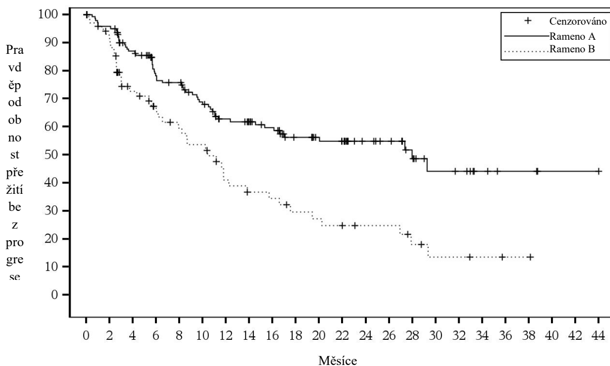
Obrázek 4: Kaplanova-Meierova křivka přežití bez progresce hodnoceného nezávislou hodnoticí komisí (populace ITT)
