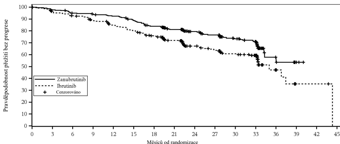
Obrázek 2: Kaplanova-Meierova křivka přežití bez progresse podle nezávislého centrálního hodnocení (ITT) (datum ukončení sběru údajů 8. srpna 2022)
