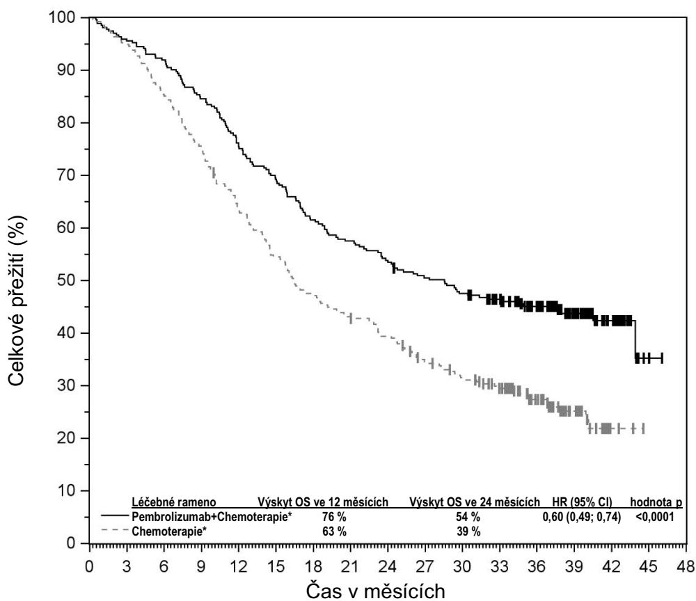
Obrázek 48: Kaplanova-Meierova křivka celkového přežití podle léčebného ramene ve studii KEYNOTE-826 u pacientek s expresí PD-L1 (CPS \geq 1 )
