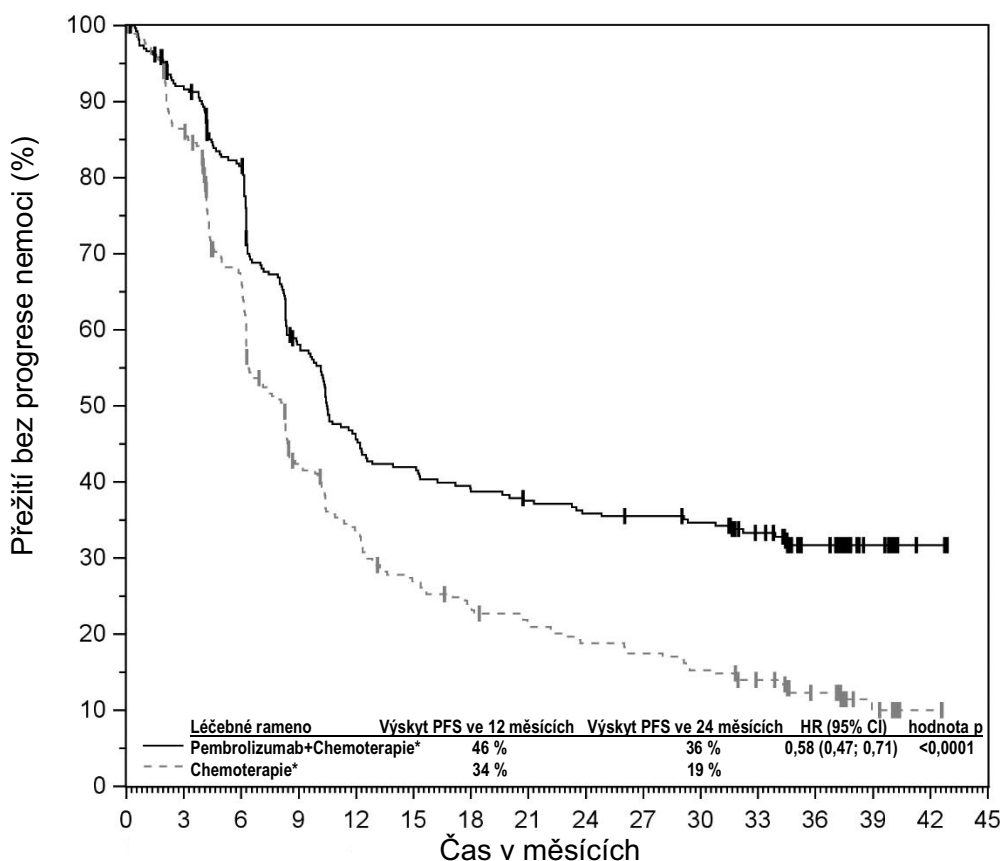
Obrázek 49: Kaplanova-Meierova křivka přežití bez progresce nemoci podle léčebného ramene ve studii KEYNOTE-826 pacientek s expresí PD-L1 (CPS \geq 1)
