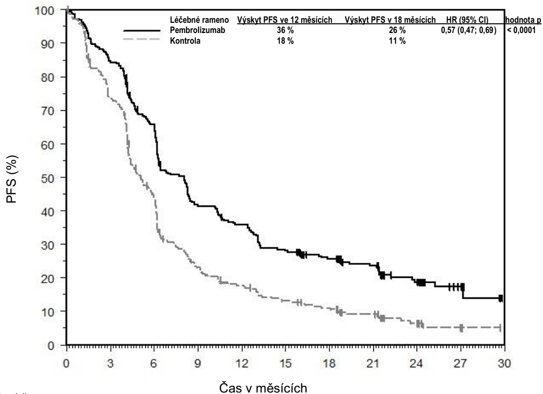
Obrázek 17: Kaplanova-Meierova křivka přežití bez progresce nemoci ve studii KEYNOTE-407
