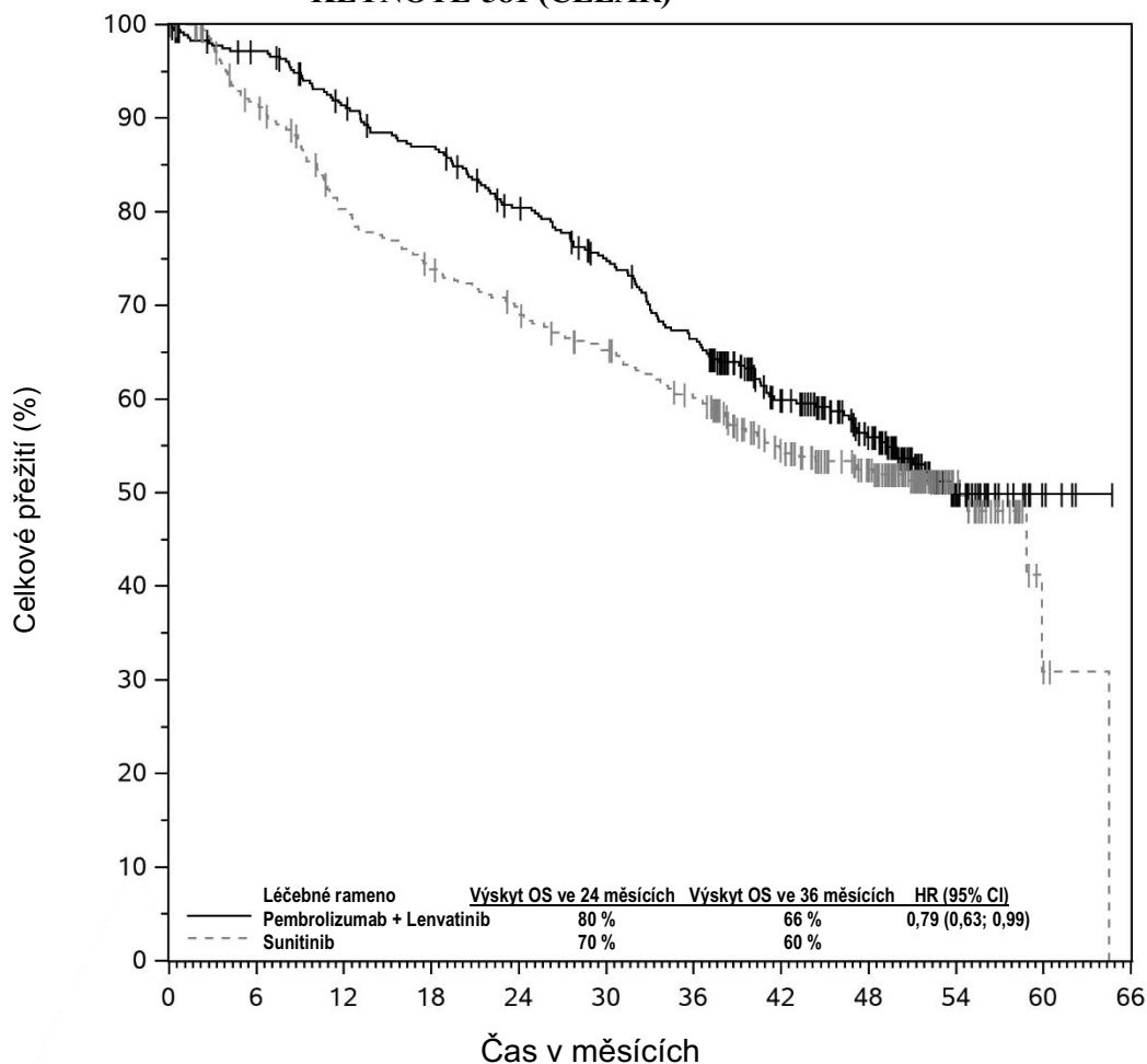
Obrázek 31: Kaplanova-Meierova křivka celkového přežití podle léčebného ramene ve studii KEYNOTE-581 (CLEAR)
