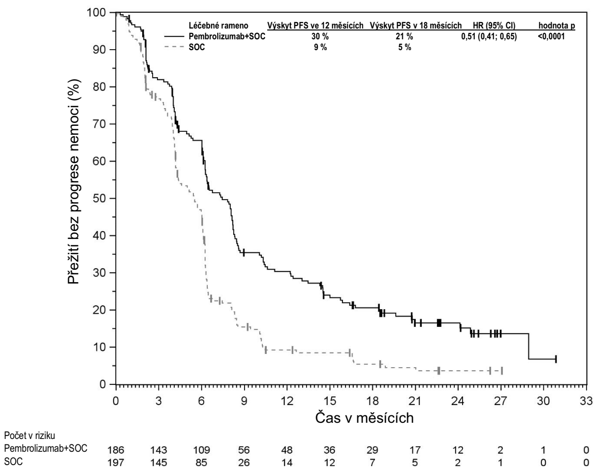
Obrázek 37: Kaplanova-Meierova křivka přežití bez progresce nemoci podle léčebného ramene ve studii KEYNOTE-590, s PD-L1 expresí (CPS ≥ 10)
