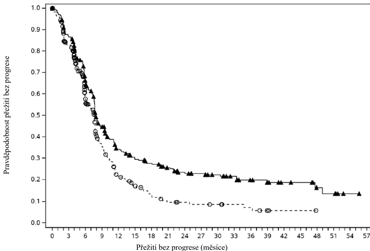
Obrázek 23: Kaplanovy-Meierovy křivky pro PFS (CA209901)
